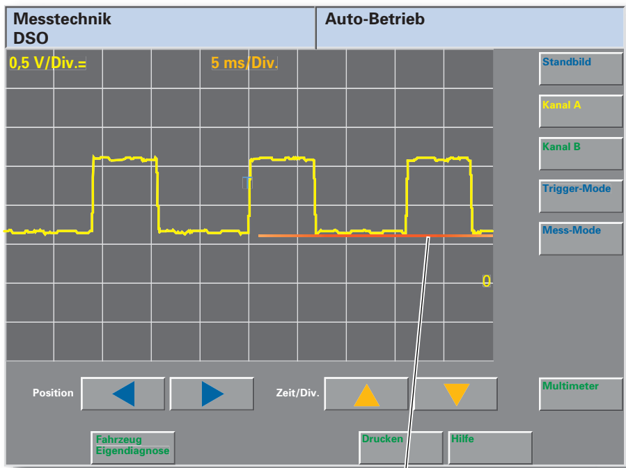
Spannungspiegel bei Fahrgeschwindigkeit 0 km/h
