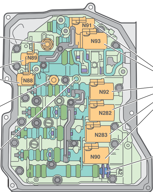
Ansicht des Schieberkastens von unten
