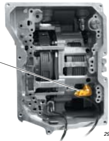
Getriebeansicht von unten
