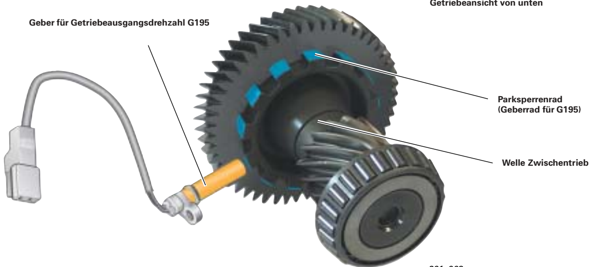
Getriebeansicht von unten
