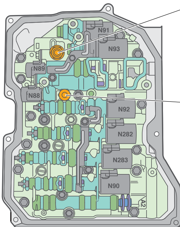
Ansicht Schieberkasten, Getriebe von unten
