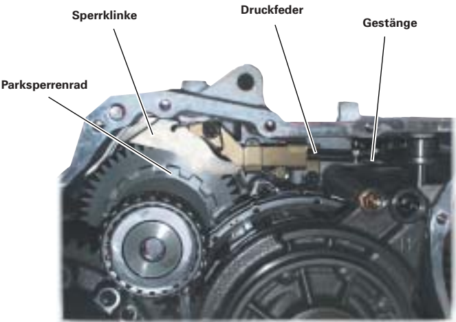
Stellung „Parksperr eingerastet“
