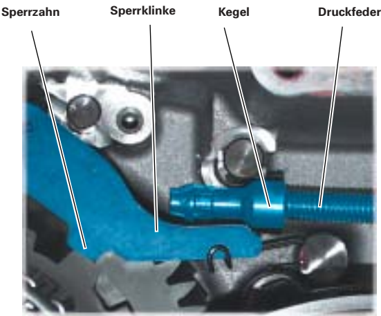
Stellung „Druckfeder vorgespannt“
