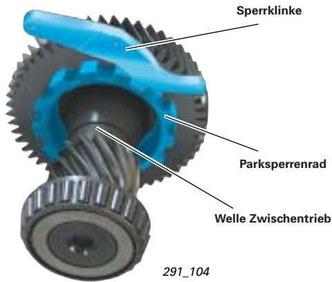
Stellung „Parksperr eingerastet“
