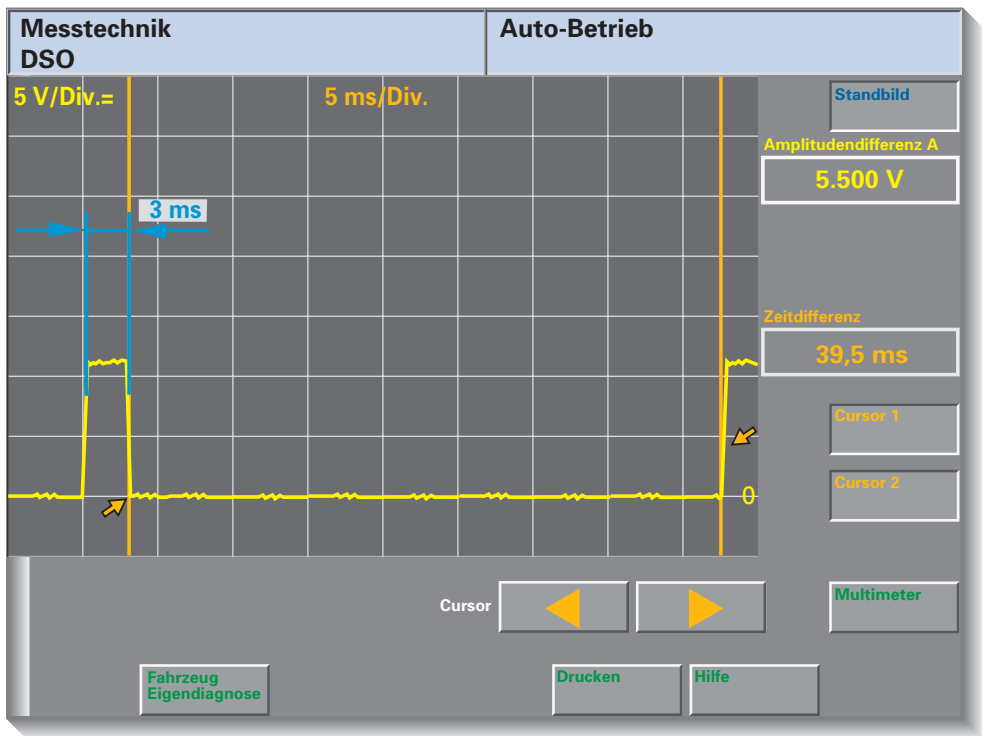
DSO-Bild – Signal vom F189, Wählhebel in P, R, N, D oder S
